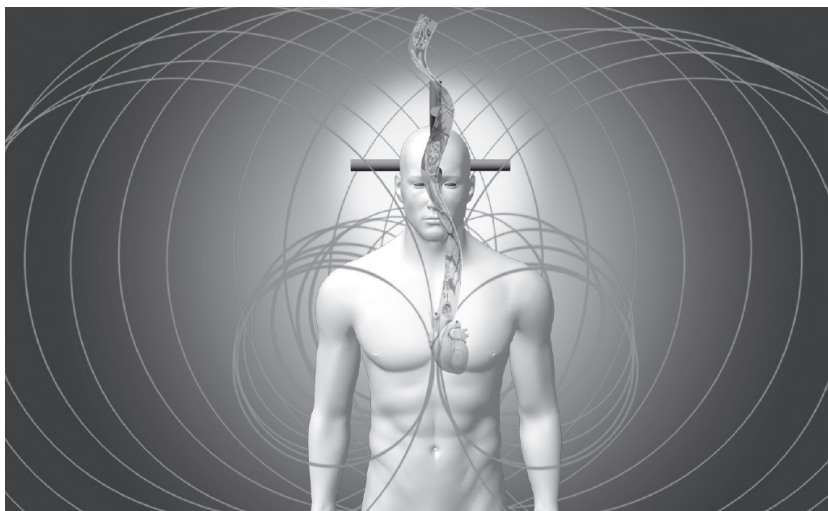
Тор сердца
